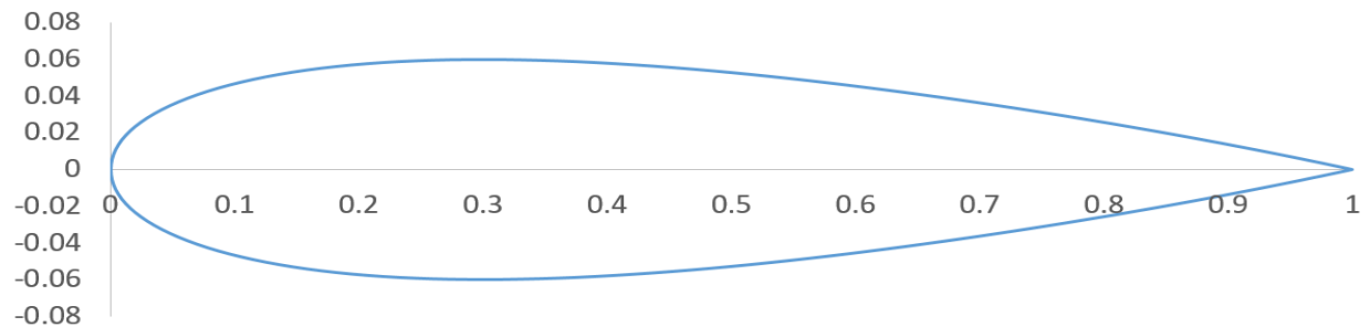
Fig. 1: NACA 0012 geometry
