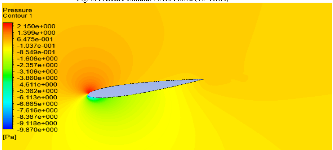
Fig. 9. Pressure Contour NACA 0012 (-10° AOA)
