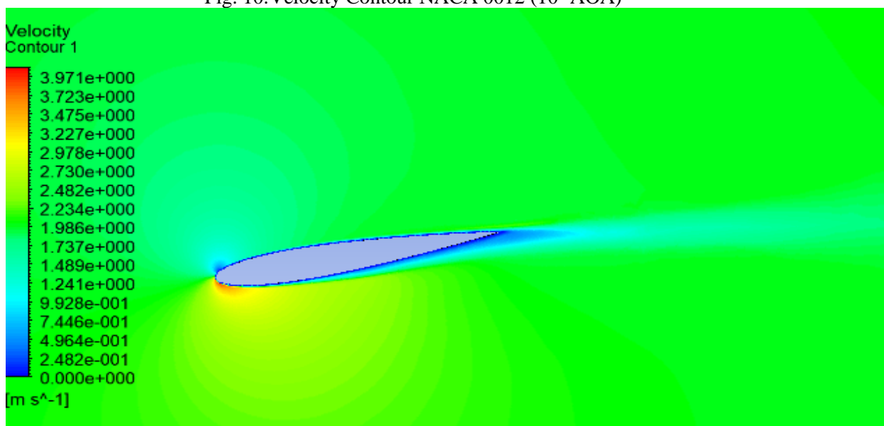
Fig. 11. Velocity Contour NACA 0012 (-10° AOA)
